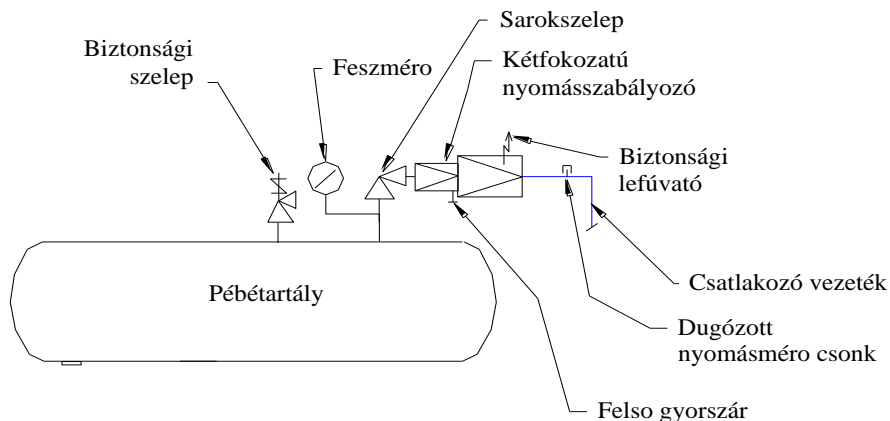
III.-8. sz. ábra Pébétartályra szerelt nyomásszabályozó max. 24 [kg/h] gázelvételre
